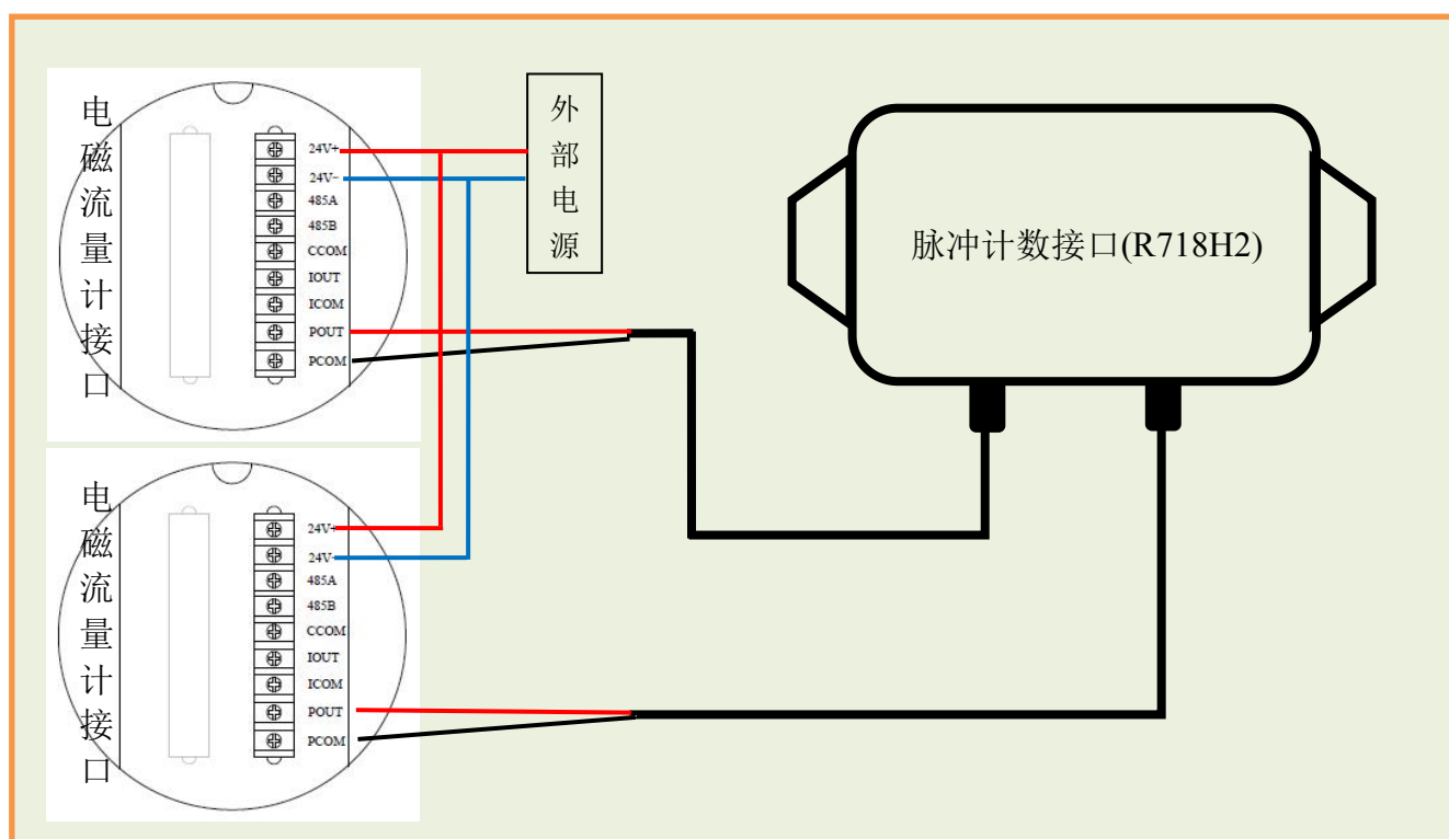
与流量计连接示意图
